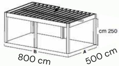
6 Piliers 500 x 800 cm
