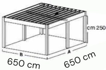
6 Piliers 650 x 650 cm
