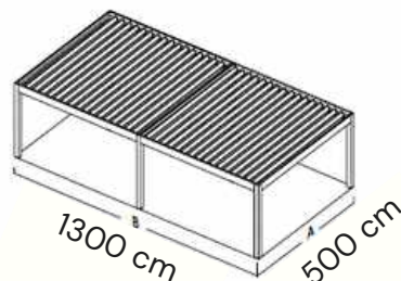
6 Piliers 1300 x 500 cm
