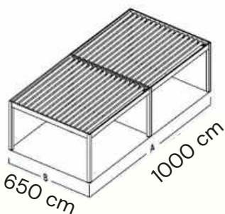
6 Piliers 650 x 1000 cm
